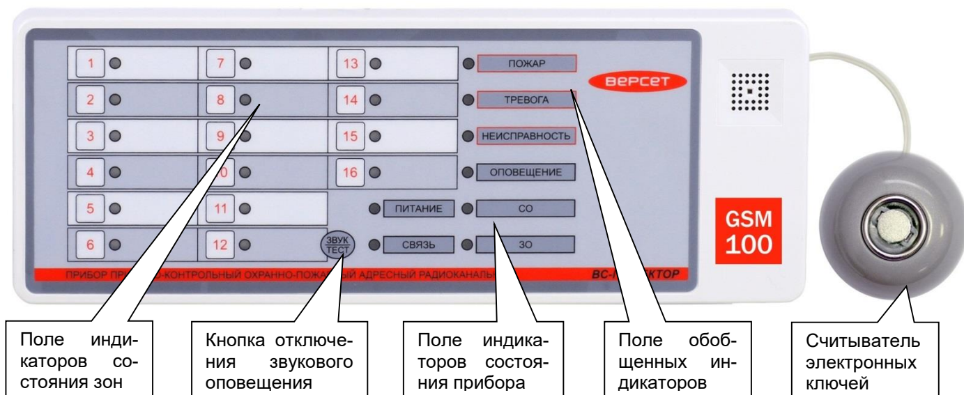
Рис. 1. Внешний вид прибора
