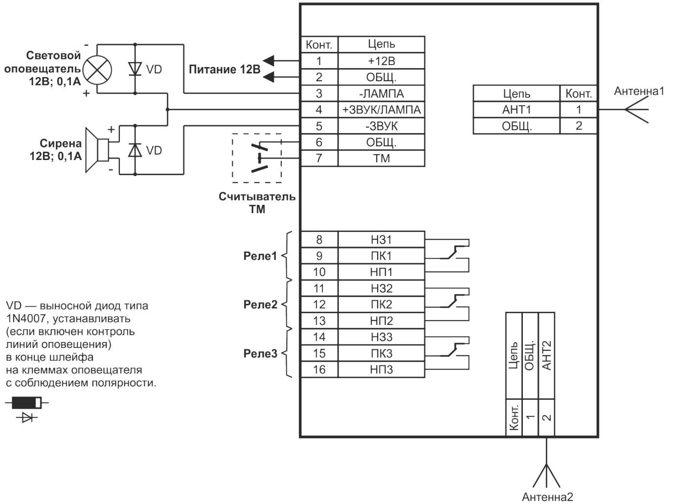
Рис.1. Схемы внешних соединений прибора ВС-ПК ВЕКТОР-АР GSM-100.
