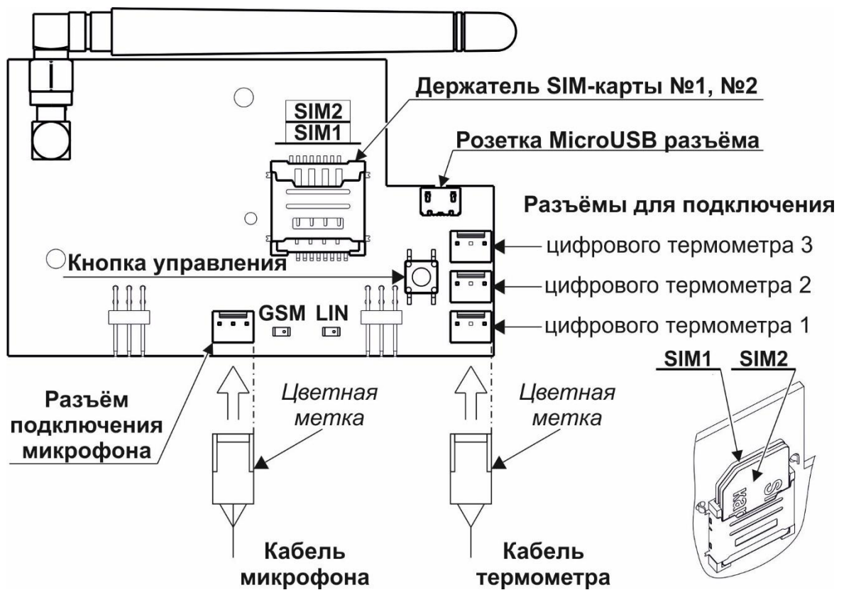
Рис.4. Внешний вид платы коммутатора прибора BC-ПК ВЕКТОР-AP GSM-100.
