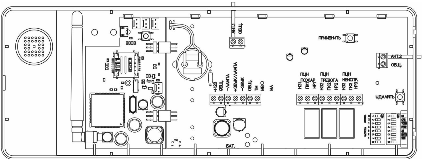
Рис.3. Внешний вид платы прибора BC-ПК ВЕКТОР-AP GSM-100.
